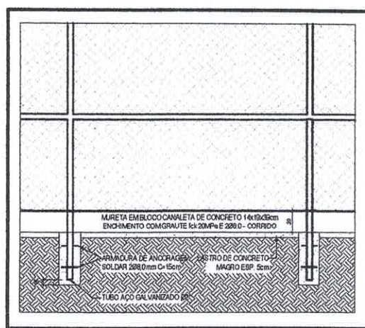
DETALHE FIXAÇÃO - ALAMBRADO E.S.C.
